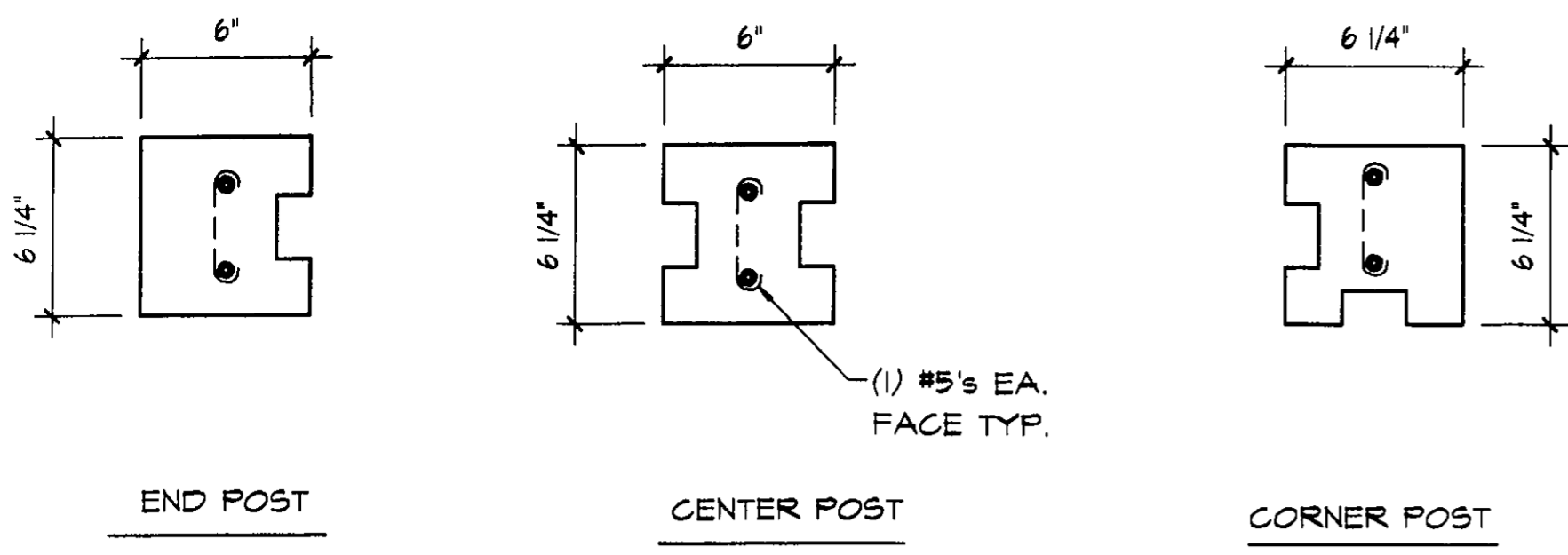
SECTIONS - POSTS SCALE: 2" = 1'-0"
